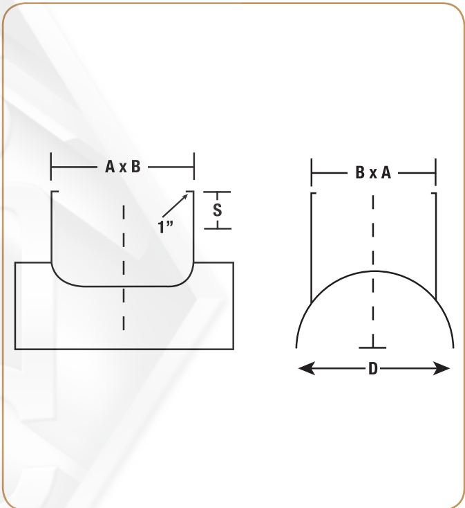
Grille Box Tap - Specify Minor Axis D
